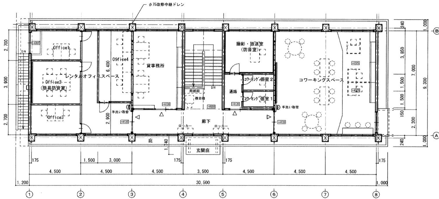
改修後2階平面図 A3, 1:200 A1, 1:100
