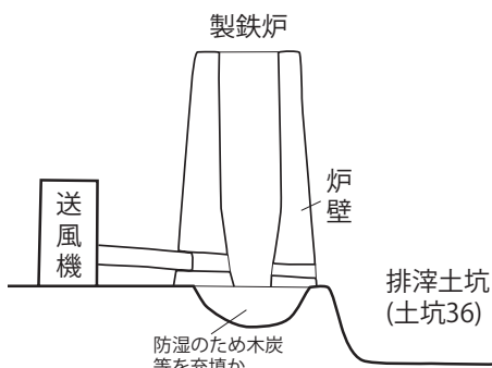
想定される製鉄炉の構造
