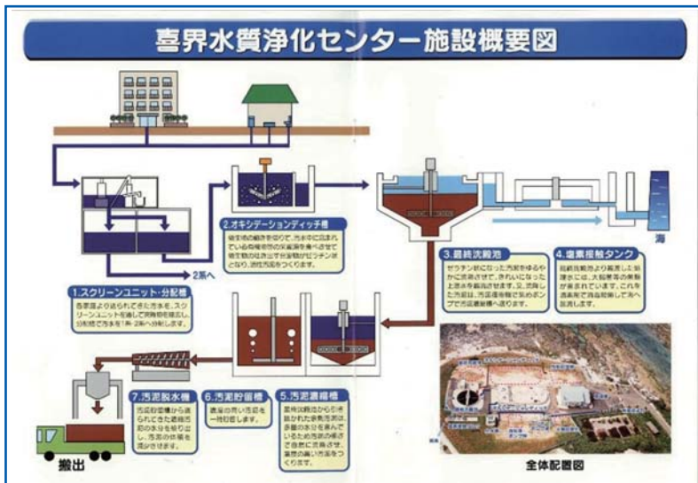
上：喜界水質浄化センター（池治） 左：喜界水質浄化センター施設概要図は島の下水処理の仕組みがよく分かる。ぜひご一読を！
